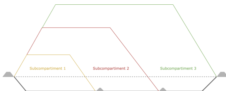
Figura 6-2 Configurația Celulei 1 din cadrul depozitului Țuțora
